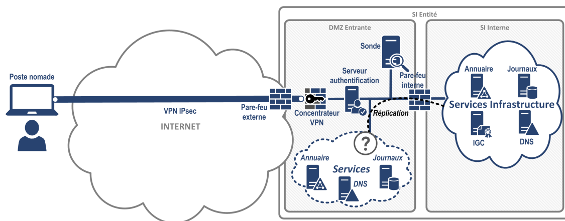
FIGURE 3.8 – Schéma global de la DMZ entrante VPN
